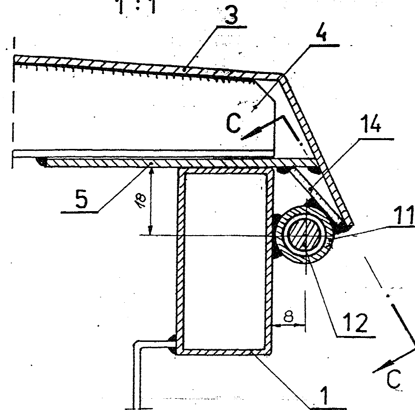
PRZEKRÓJ B-B
