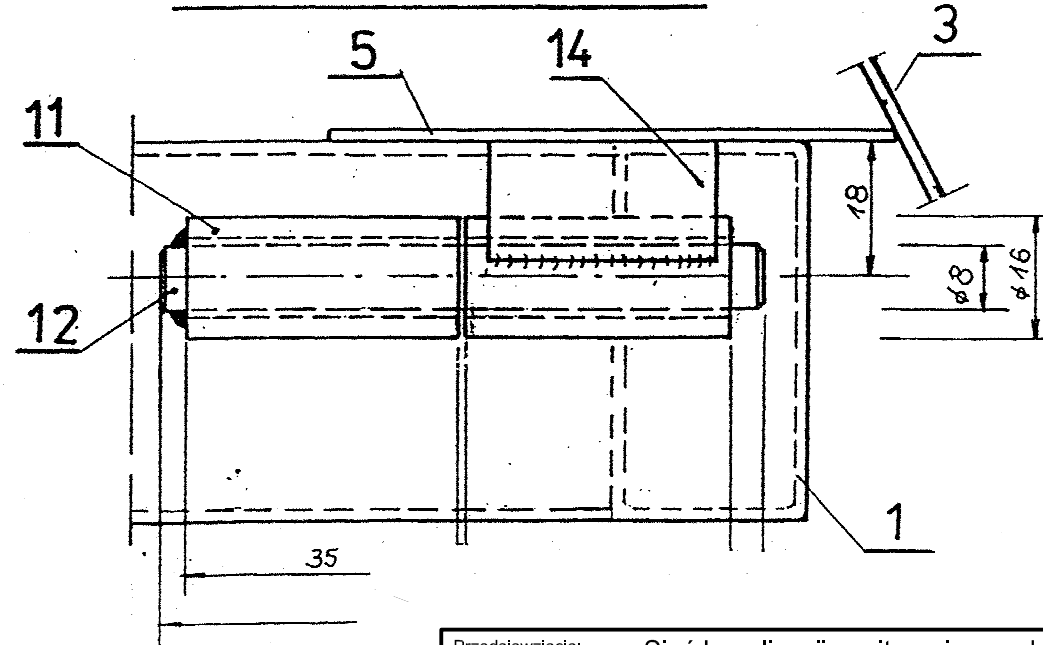
WIDOK C-C 1:1
