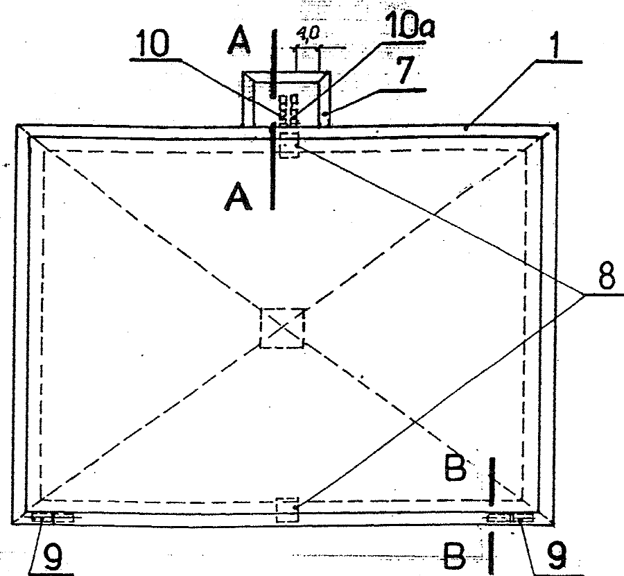
RZUT POKRYWY 1:10
