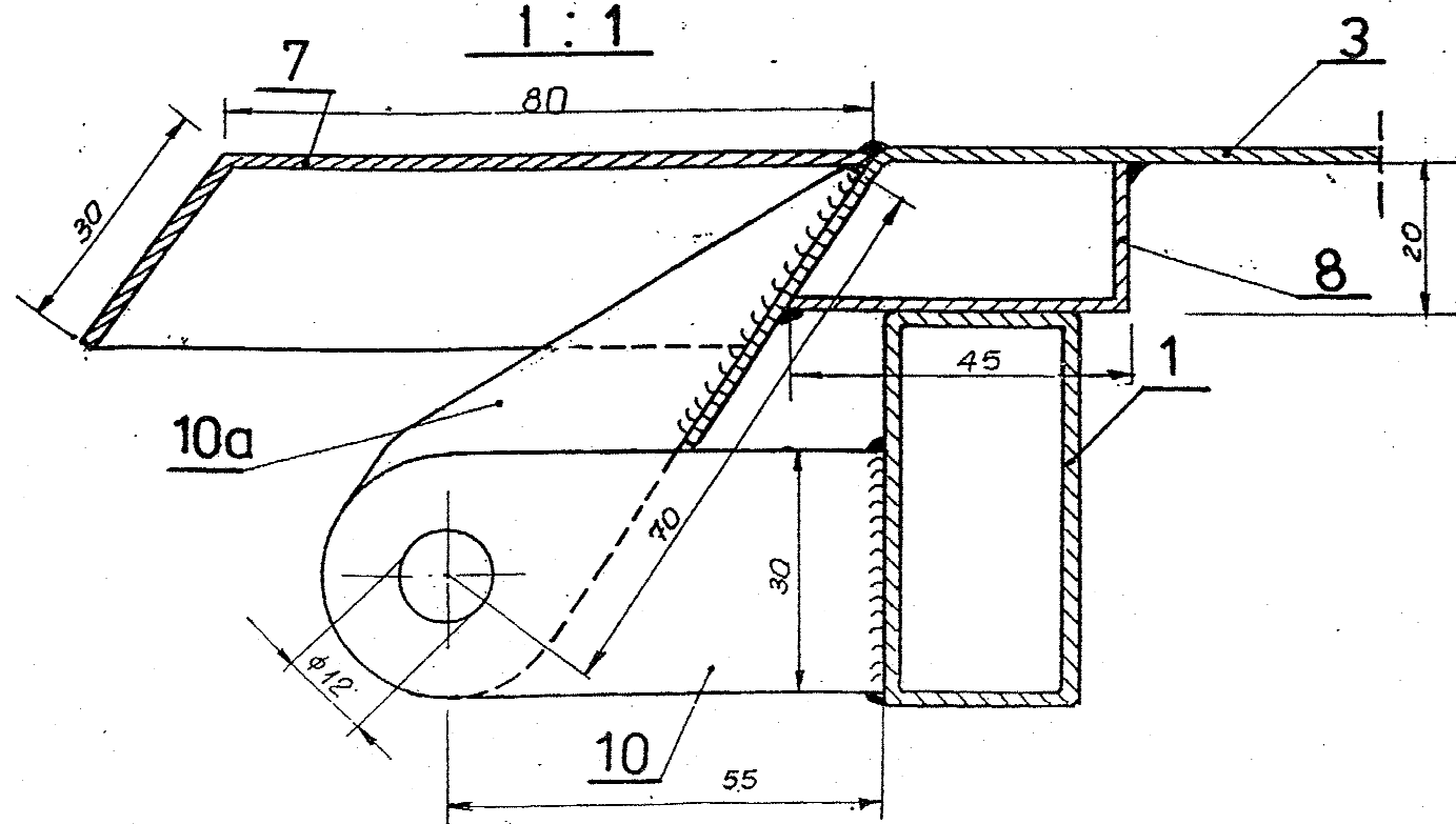
PRZEKRÓJ A-A
