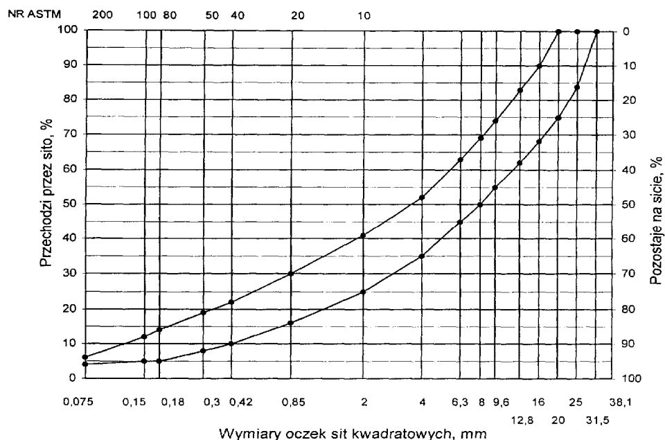
Rys. 12. Krzywe graniczne uziarnienia mieszanki mineralnej BA od 0 do 20 mm do warstwy wiążącej, wyrównawczej i wzmacniającej nawierzchni drogi o
