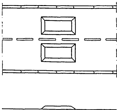
Rys. 2. Wymiary progów zwalniających wyspowych (wg [23])
